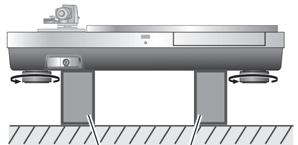
Coussin d'emballage
