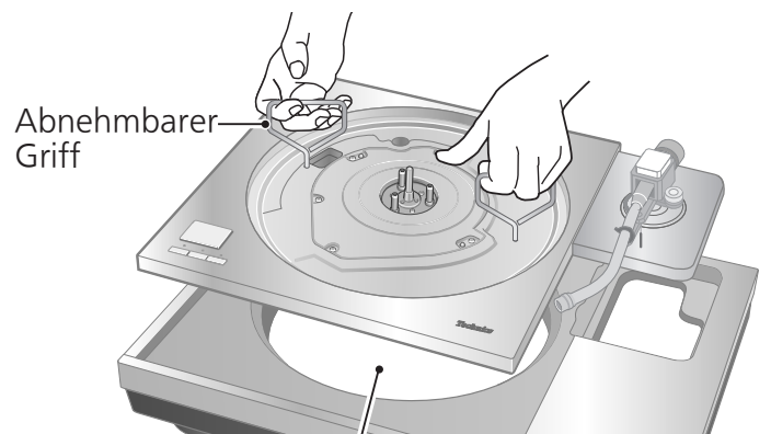
Führen Sie das Anschlusskabel des Steuergeräts durch das Loch in der Plattentellerbasis.
